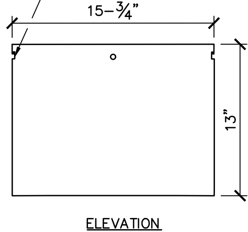
(B) CLEANOUT DOOR
